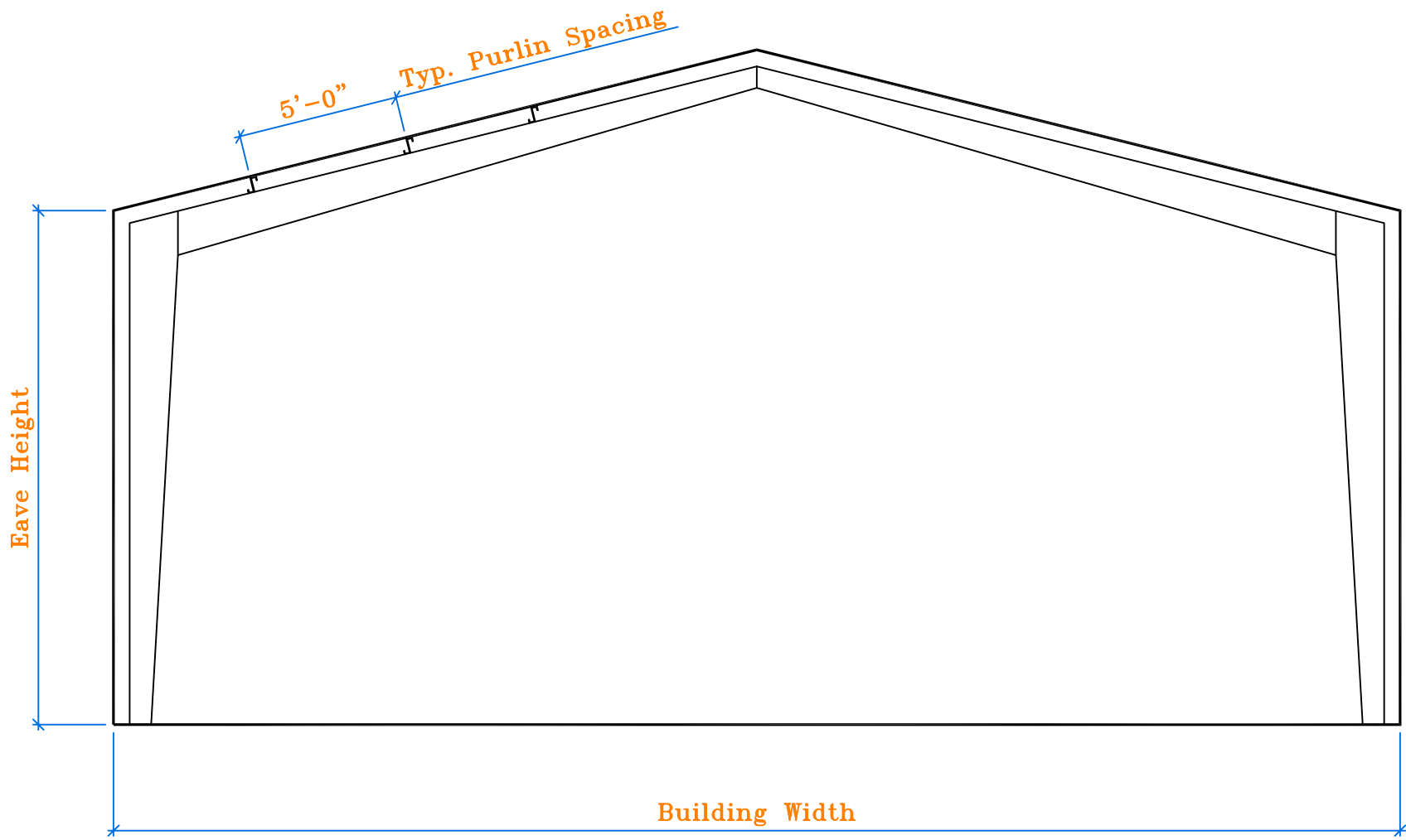
RIGID FRAME
