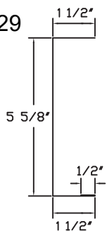
Pole Barn Eave Trim
