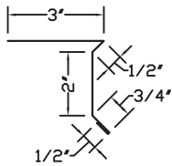
Simple Drip Edge
